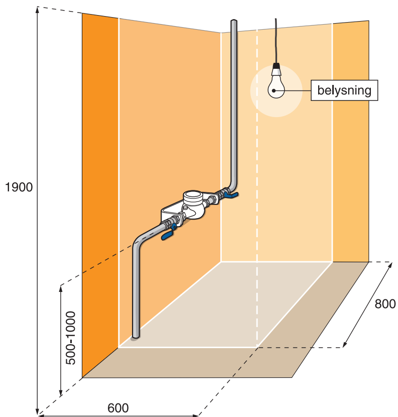
Figur 3: Placering av vattenmätare.
