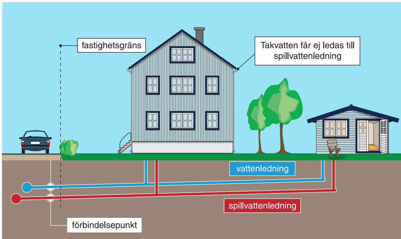
Figur 1: Servisledningens olika delar.
